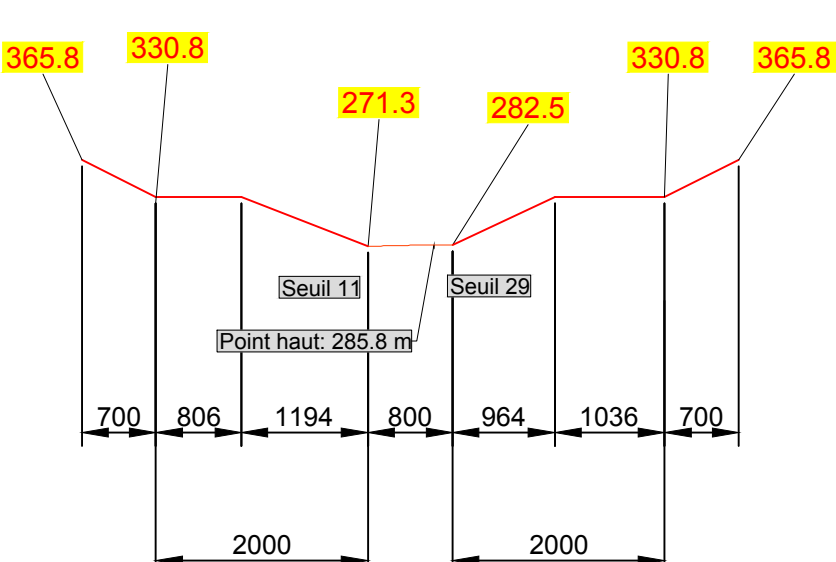
Profil en long A - A'
