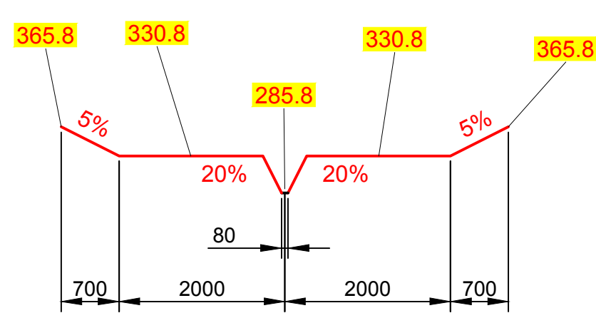
Profil en travers B - B'
